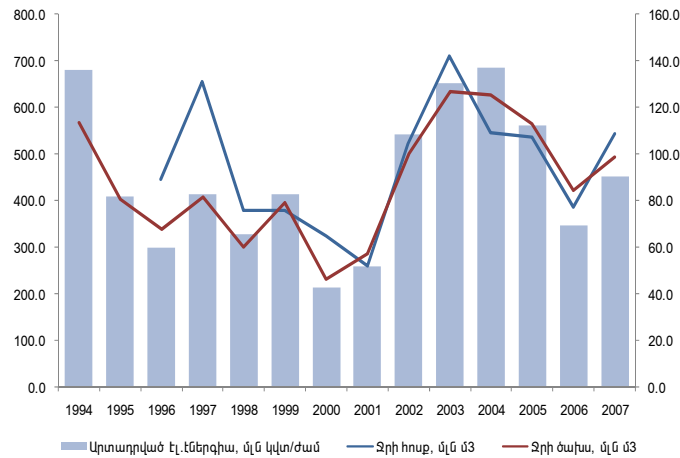
Գծանկար 3. Սարսանգ ՀԷԿ-ի հիմնական ցուցանիշները
